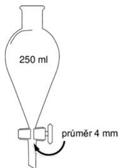
Dělicí nálevka
